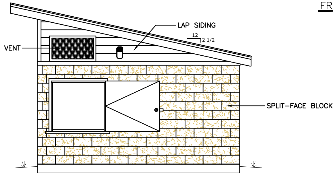
RIGHT ELEVATION
